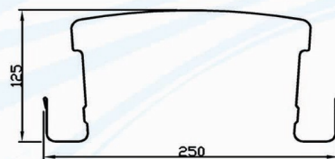
几字形栽培槽 (常用于种植番茄等作物)
